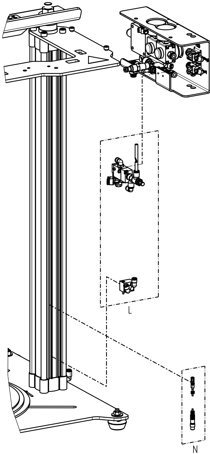
Ausbauoptionen Signal pneumatisch oder elektrisch Pneumatic or electric signal expansion option
